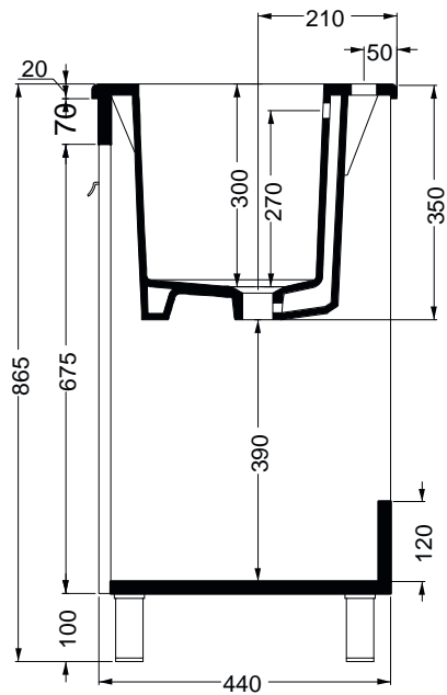
SEZIONE A-A'
