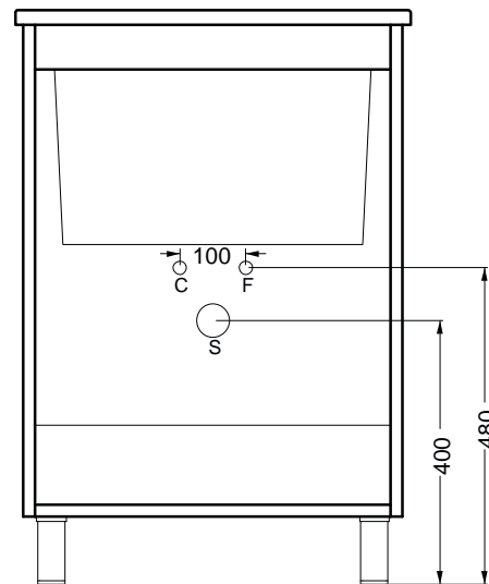
VISTA FRONTALE SENZA ANTE
