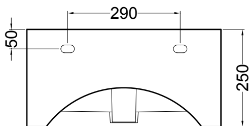
VISTA POSTERIORE
