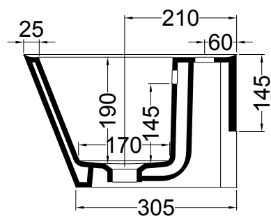
SEZIONE A-A'
